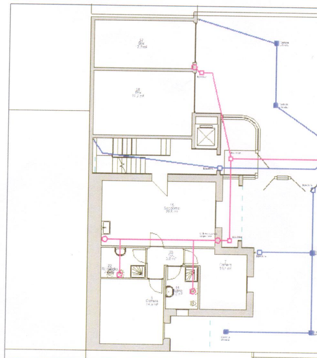
6 0 - Piano Terra - Stato modificato - Scarichi - PdR SCALE 1 : 100
